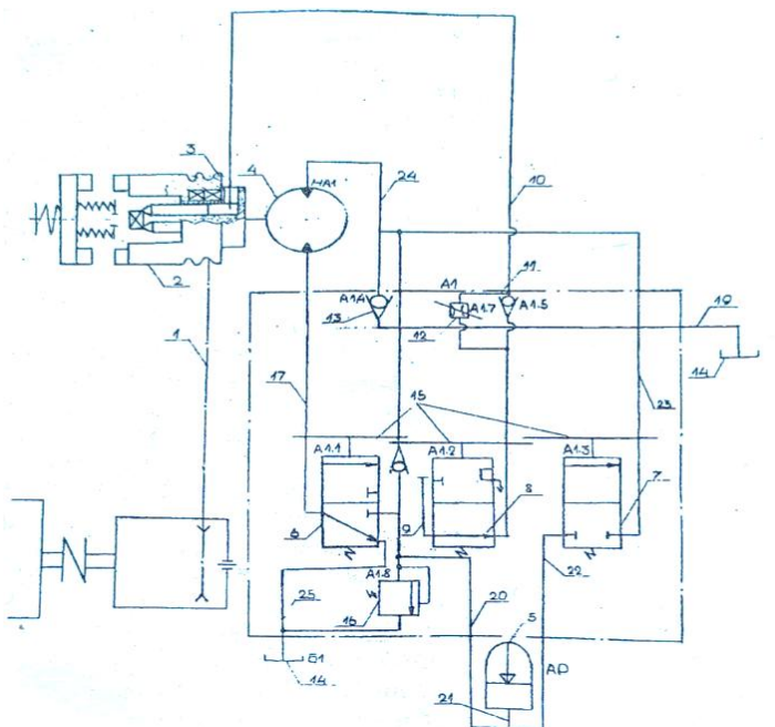
Рисунок 1 – Принципиальная схема рекуператора
